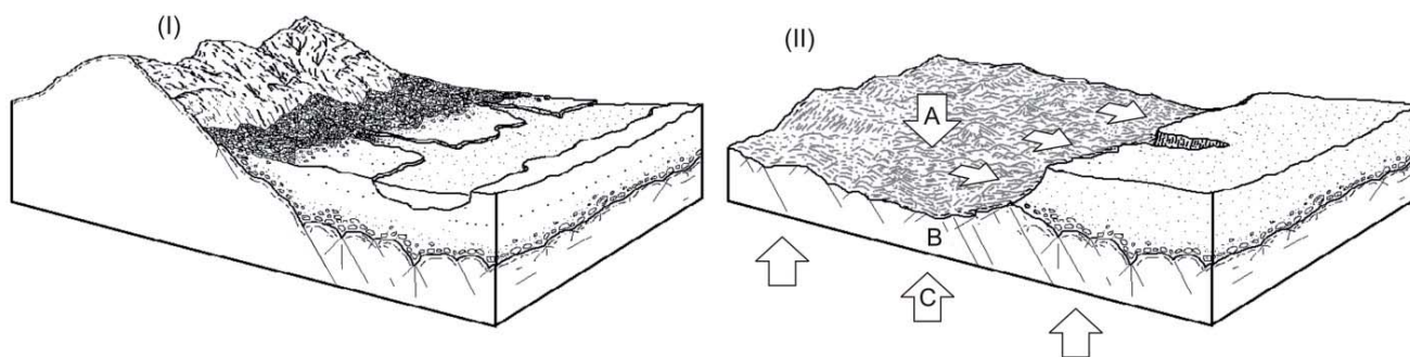
Figura 8 - Modelo de inversão do relevo segundo processos estruturais/denudacionais. (A) Erosão diferencial do embasamento, (B) Reativação frágil (compressional) ao longo da ZCP, (C) Epirogênese (Underplating).
